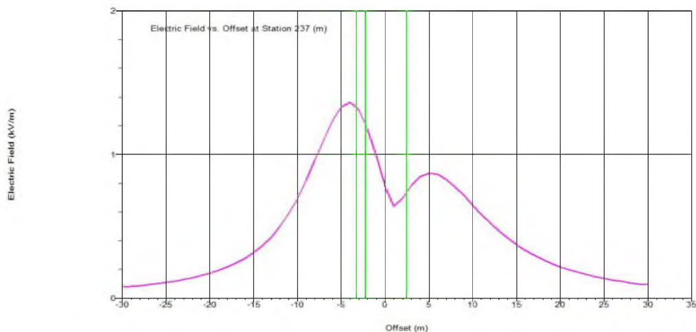
Графикон 1. Максимална јачина електричног поља
