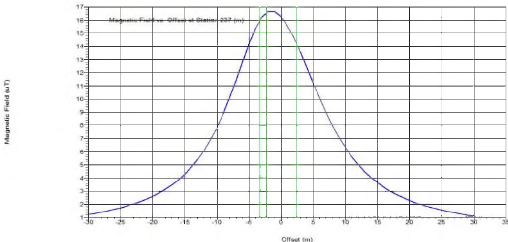
Графикон 2. Максимална јачина магнетног поља
